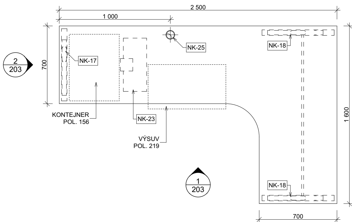
POLOŽKA 203 - KANCELÁŘSKÝ STŮL L, PRAVÝ
