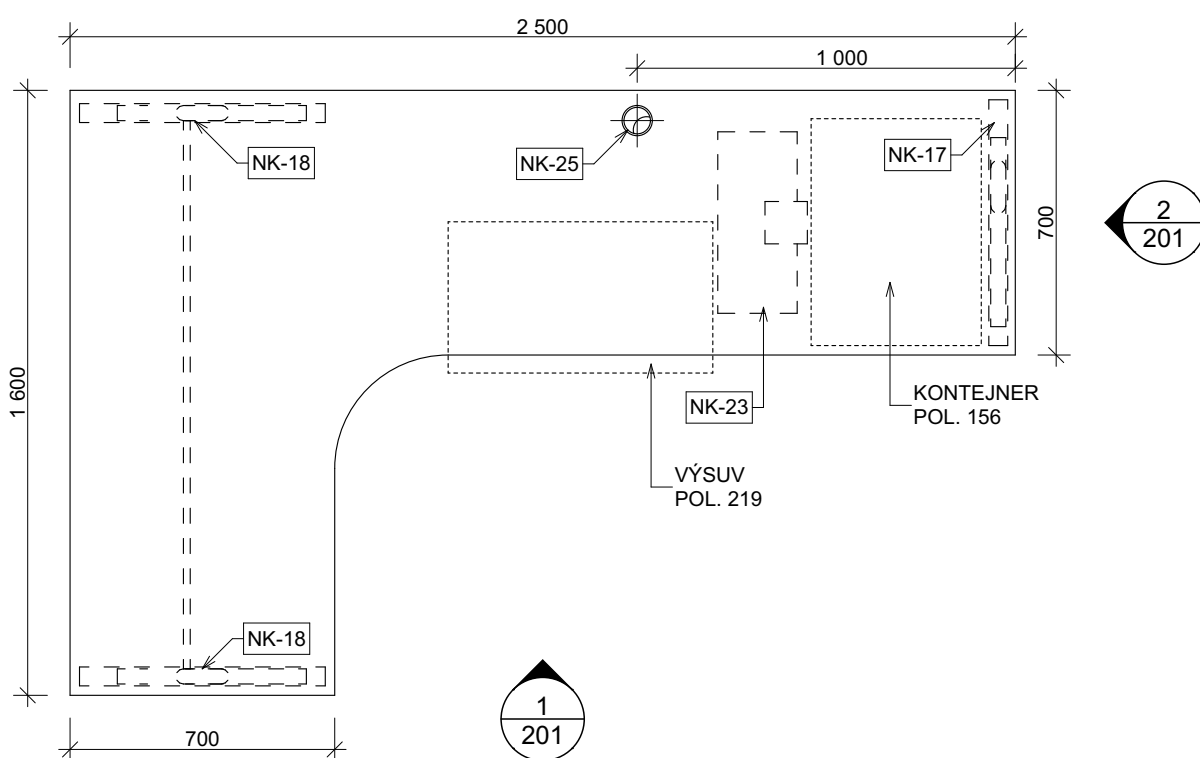
POLOŽKA 201 - KANCELÁŘSKÝ STŮL L, LEVÝ
